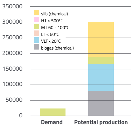
Energievraag en potentiële energieproductie bij de rwzi van Amersfoort
