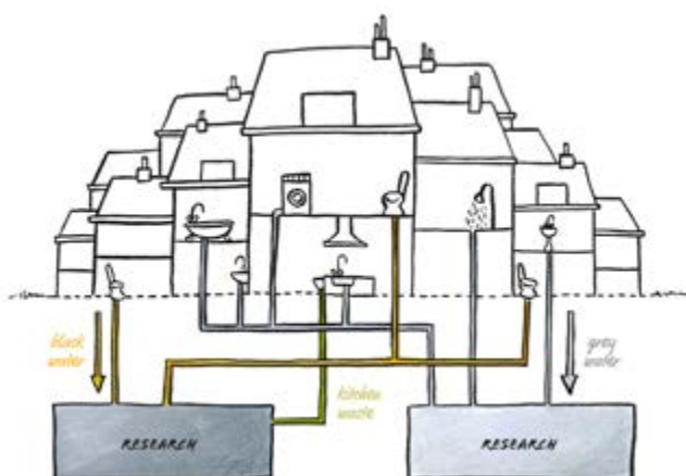
Afb. 4.6 Schematische weergave van het concept van een gescheiden afvalwateropvangstelsel
