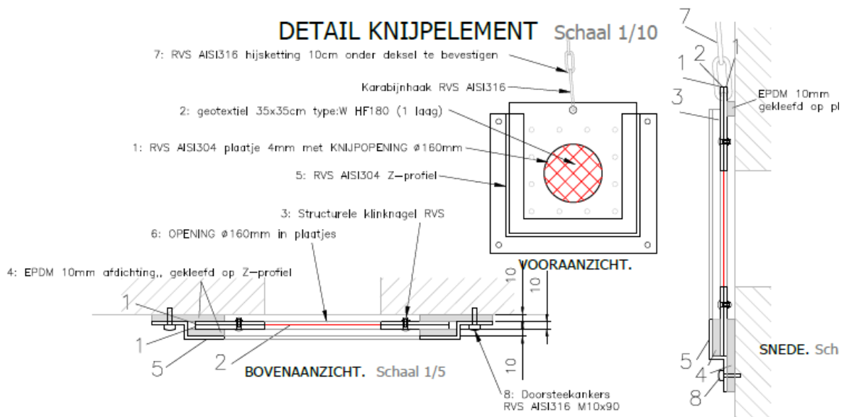
Figuur 5: Principe van een knijopening met geotextiel (bron: Studiebureau Jonckheere)
